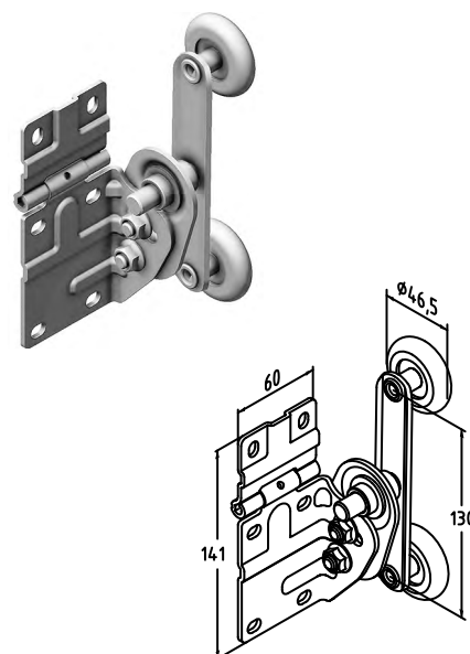
Кронштейн боковой для промышленных ворот
