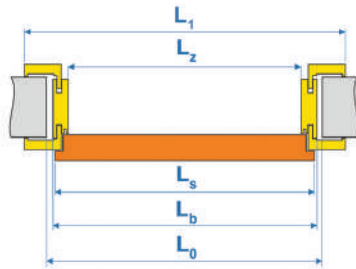
З коробкою Eco-Fit
