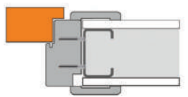
Монтаж в гіпсокартонну стіну за допомогою болтів
