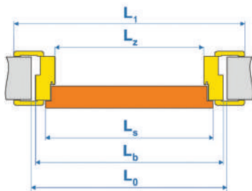
З коробкою CLASSIC
