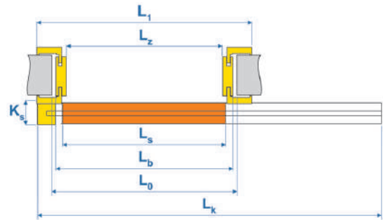
Розсувна система Eco-SLIDE з дверною коробкою Eco-Fit
