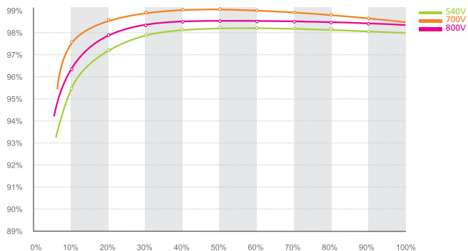
Эффективность MAX 80KTL3 LV
