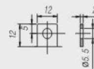
Terminal F2
