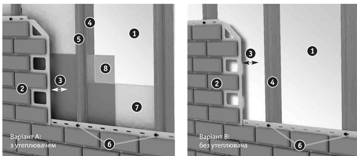
1 – стіна будинку, 2 – фасадна панель, 3 – вентиляований зазор, 4 – рейка 50х50 мм, 5 – рейка 25х25 мм, 6 – шуруп, 7 – утеплювач, 8 – гідроізолююча плівка
