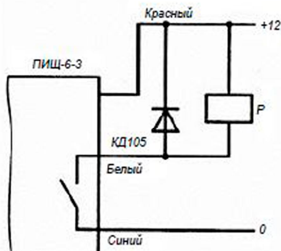
Схема подключения к индуктивной нагрузке при использовании одного источника питания.
