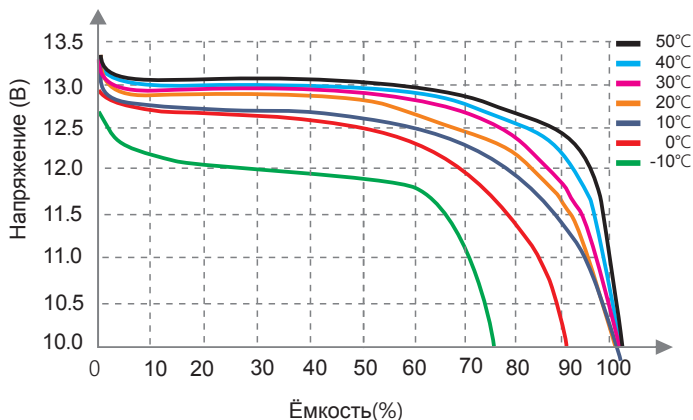
Характеристика разряда при разных температурах
