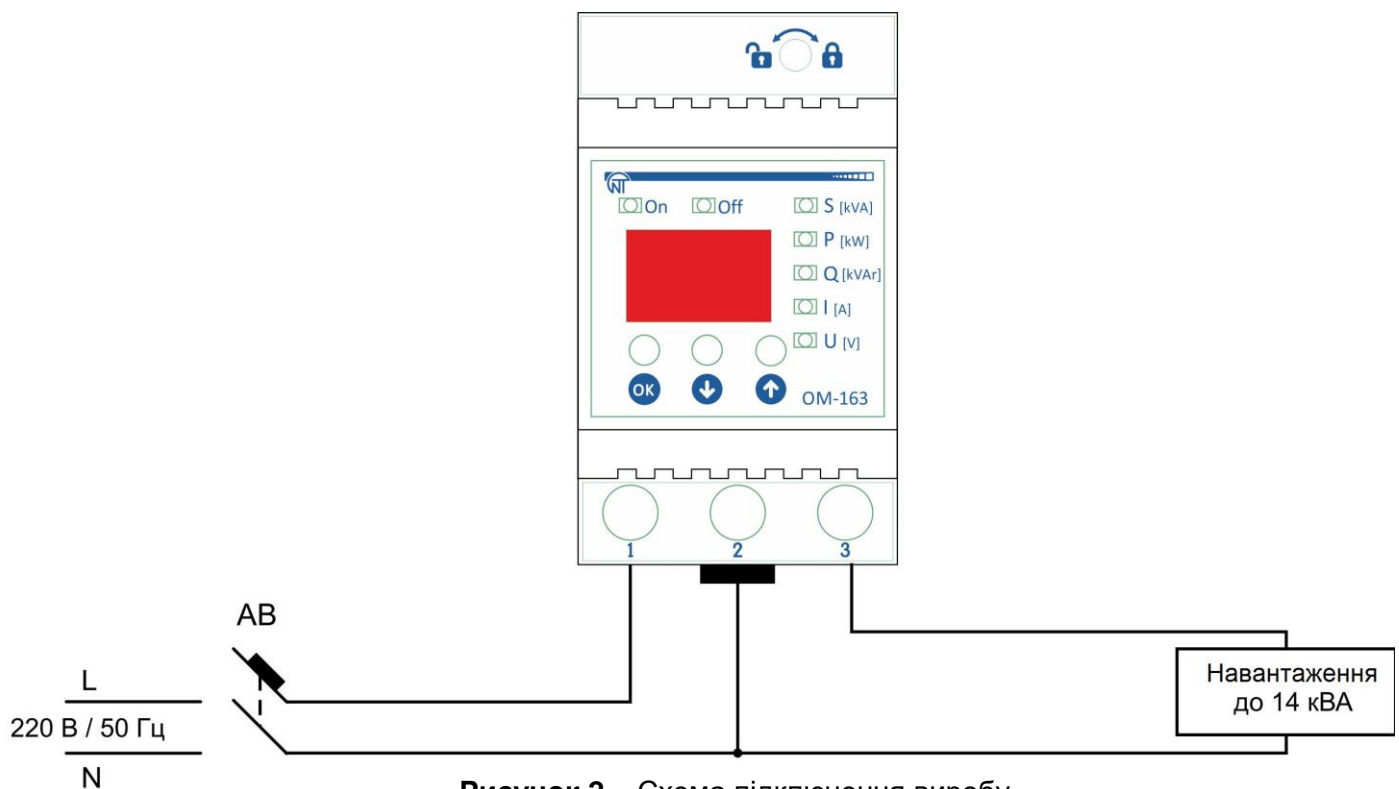
Рисунок 2 – Схема підключення виробу
