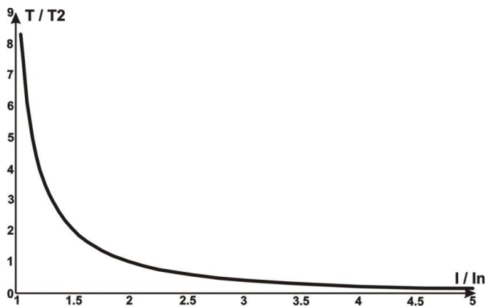
Рисунок 6 – Струмо-часова характеристика
