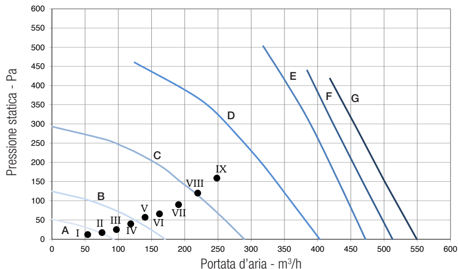
Fig. 6.g Curva di immissione in accordo al Reg. 1253/2014 (ErP). Prodotto testato senza filtro F7.
