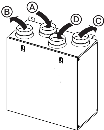
Fig. 3.a Connessioni orientamento SX e DX - QR280A.
