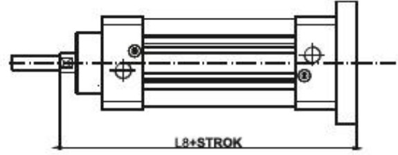
ARKA FLANŞ BAĞLANTI / REAR FLANGE MOUNTING
