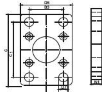
FB:FLANŞ BAĞLANTI / FLANGE MOUNTING
