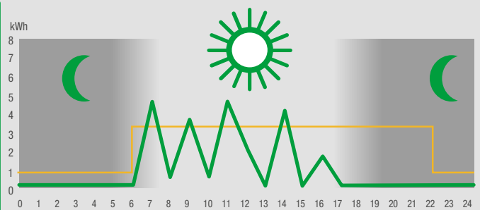
Energy consumption with a conventional cooling system (simulation) Energieverbrauch mit einem konventionellen Kühlsystem (Simulation) Consommation d'énergie avec un système de refroidissement conventionnel (simulation)
