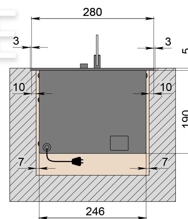
Монтаж заподлицо
