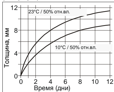
Граф. 1: Скорость отвердевания Sikaflex®-296
