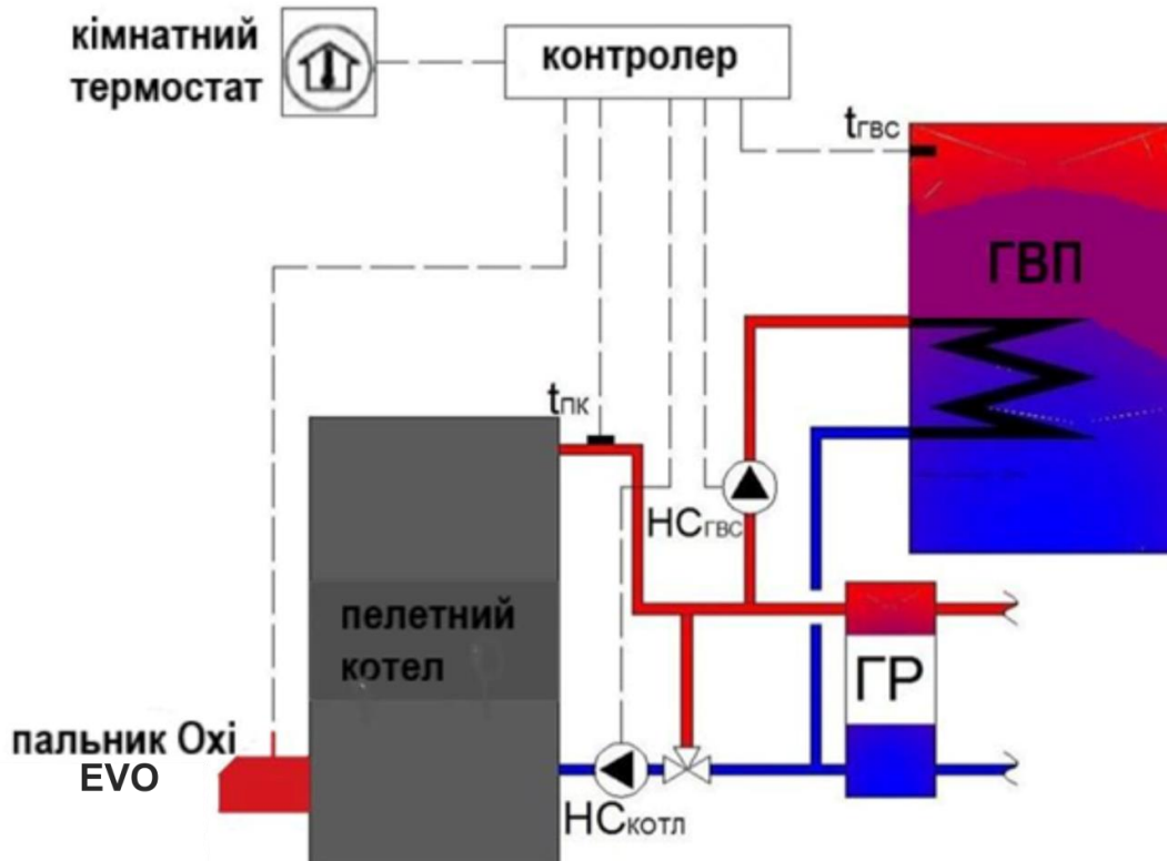
Малюнок 7. Принципова схема №1
