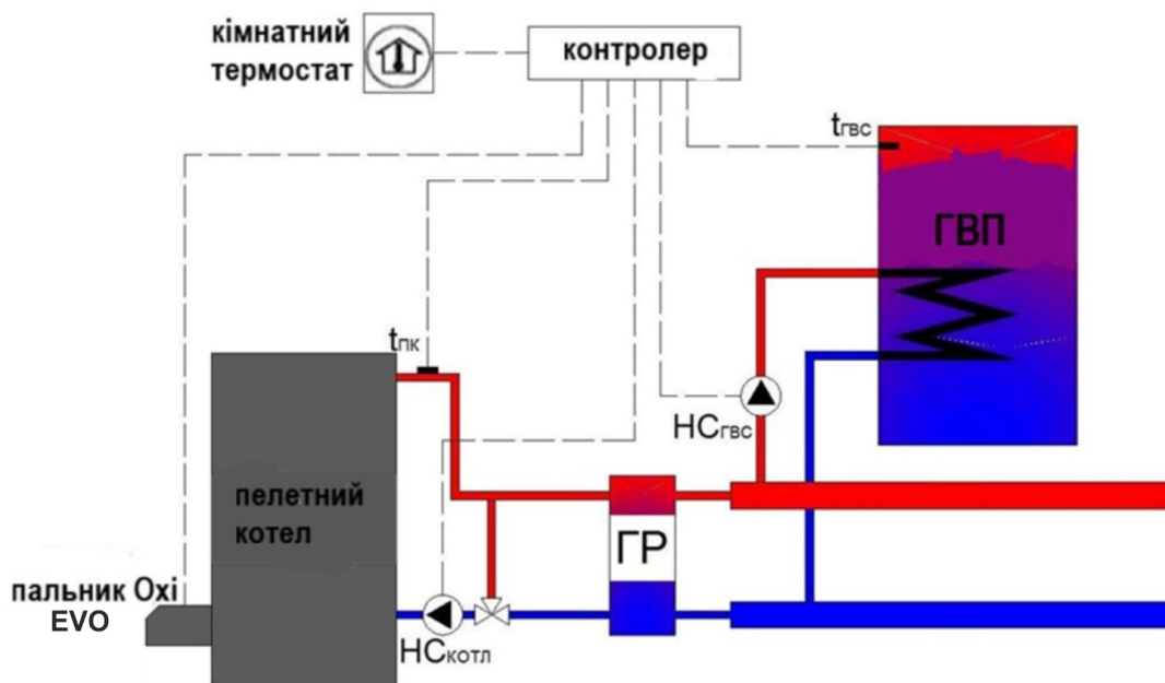
Малюнок 8. Принципова схема №2
