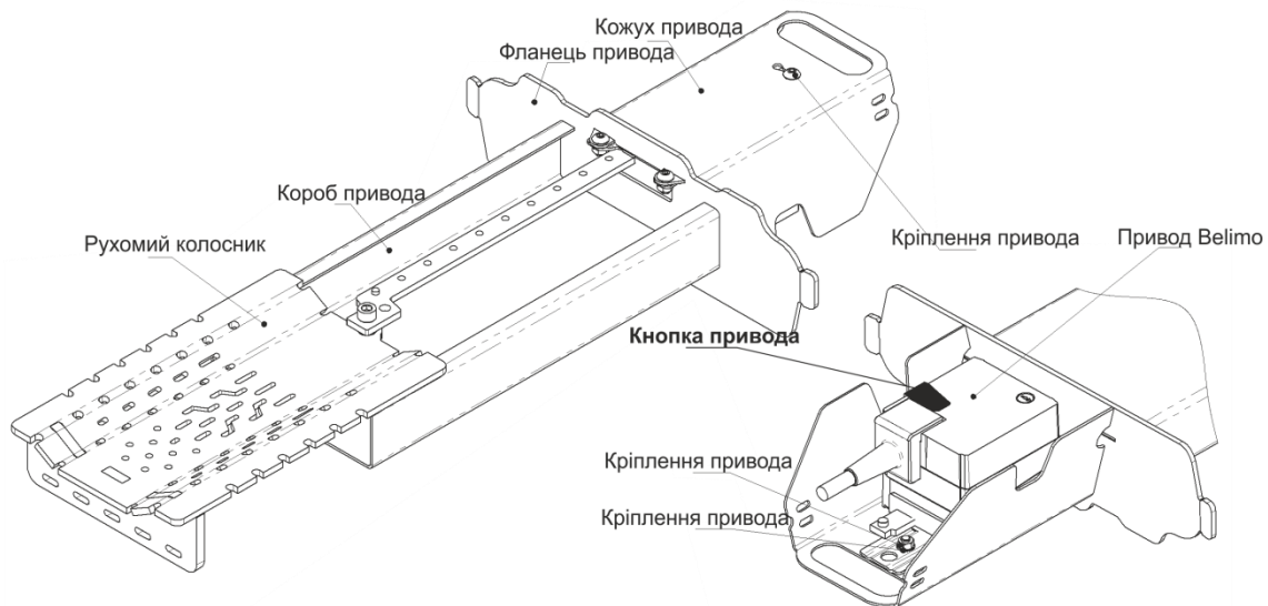
Малюнок 12. Устрій колосникового блоку
