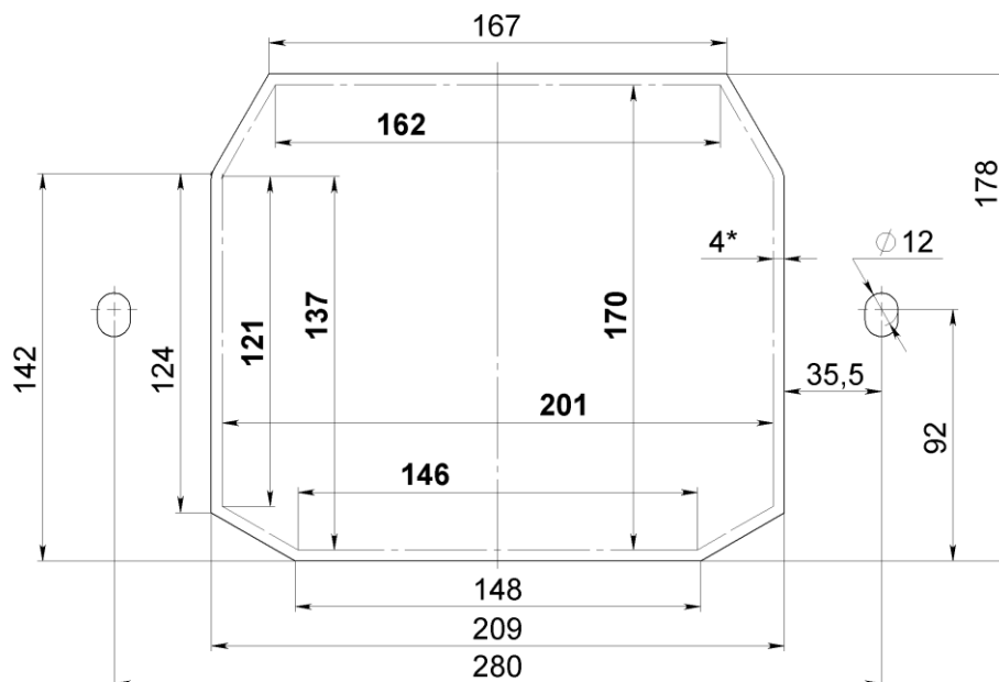
Малюнок 4. Габаритні розміри монтажного отвору в дверцях котла
