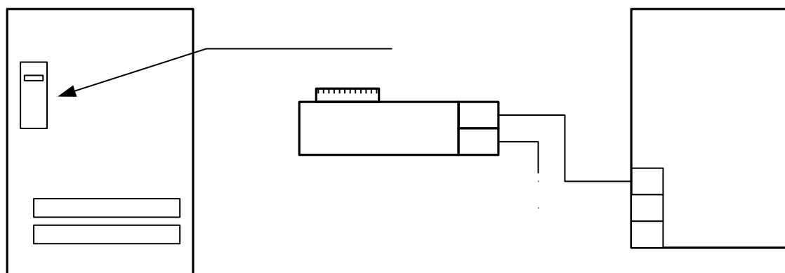
Малюнок 5 – підключення контролера до мережі змінного струму
