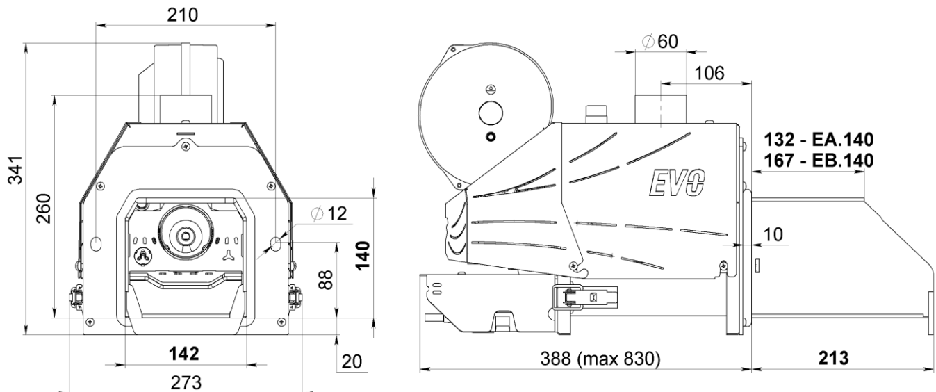
Малюнок 1. Габаритні розміри пальників OXI EVO 20-30 кВт з шамотованою камерою згоряння.
