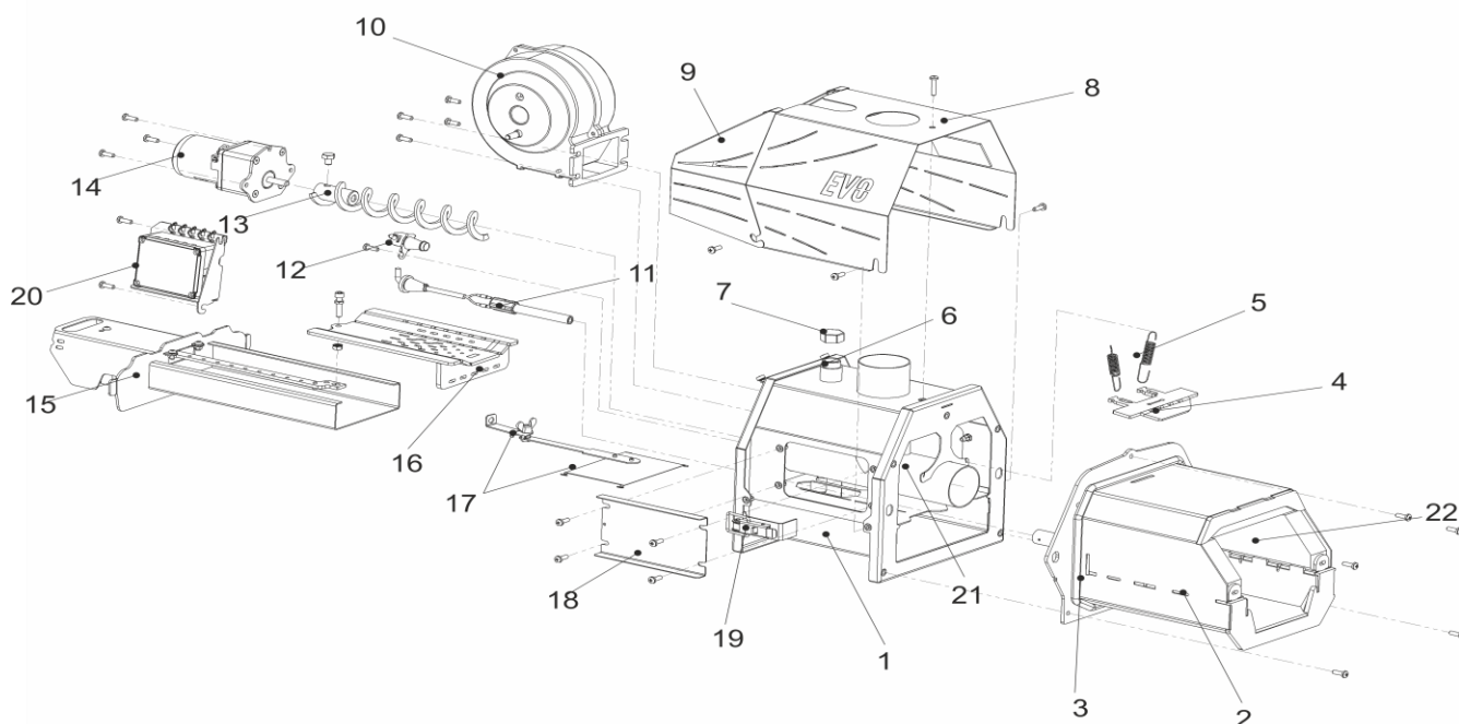
Малюнок 2. Елементи пальника OXI EVO
