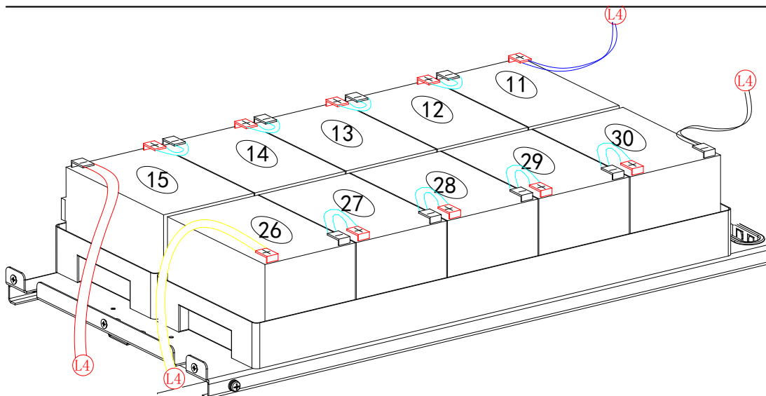
Рис.6-2-4 Соединение Яруса 3
