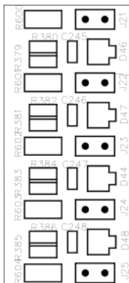
Рис.5-12 Перемычки на плате управления (PS1203_CT1)
