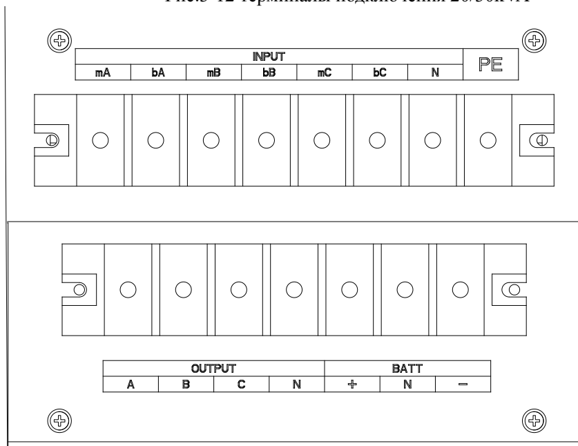
Рис.3-13 терминалы подключения 40kVA
