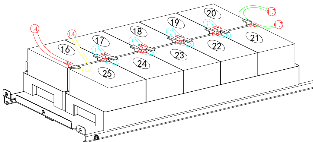
Рис.6-2-5 Соединения Яруса 4
