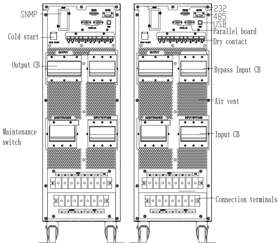
Рис. 2-13 ИБП 40кВа, внешние батареи, задняя панель
