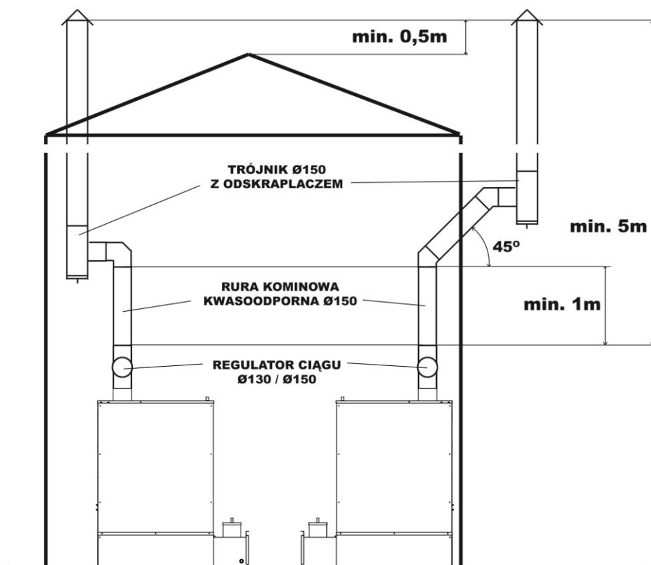
Рис. 4. Дымоходная система
