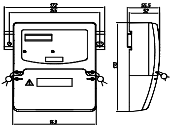
Рисунок 1 - Загальний вигляд лічильника ЦЗ6804-У у корпусі Р32
