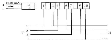
Рисунок 2 - Схема підключення лічильника
