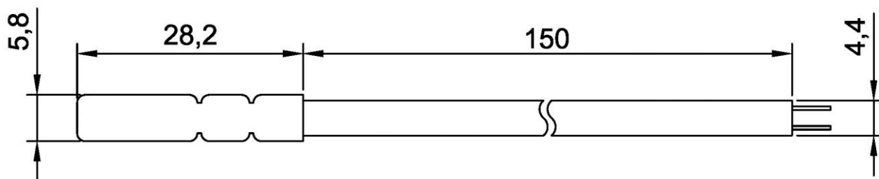
Рисунок 2 - Внешний вид и габаритные размеры
