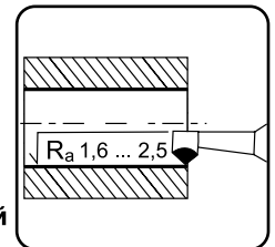
Растачивание отверстий
