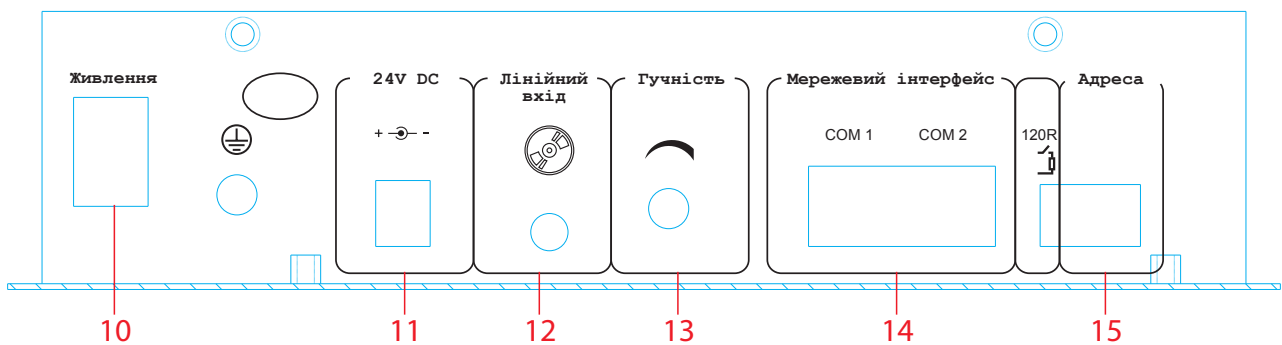
Мал. 2.2 Мікрофонна консоль ITC VA-16ZRM (задня панель)
