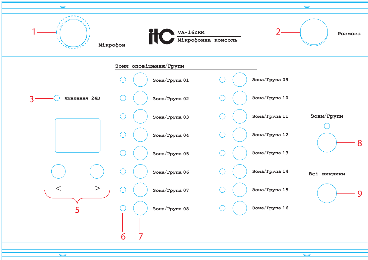
Мал. 2.1 Мікрофонна консоль ITC VA-16ZRM (передня панель)
