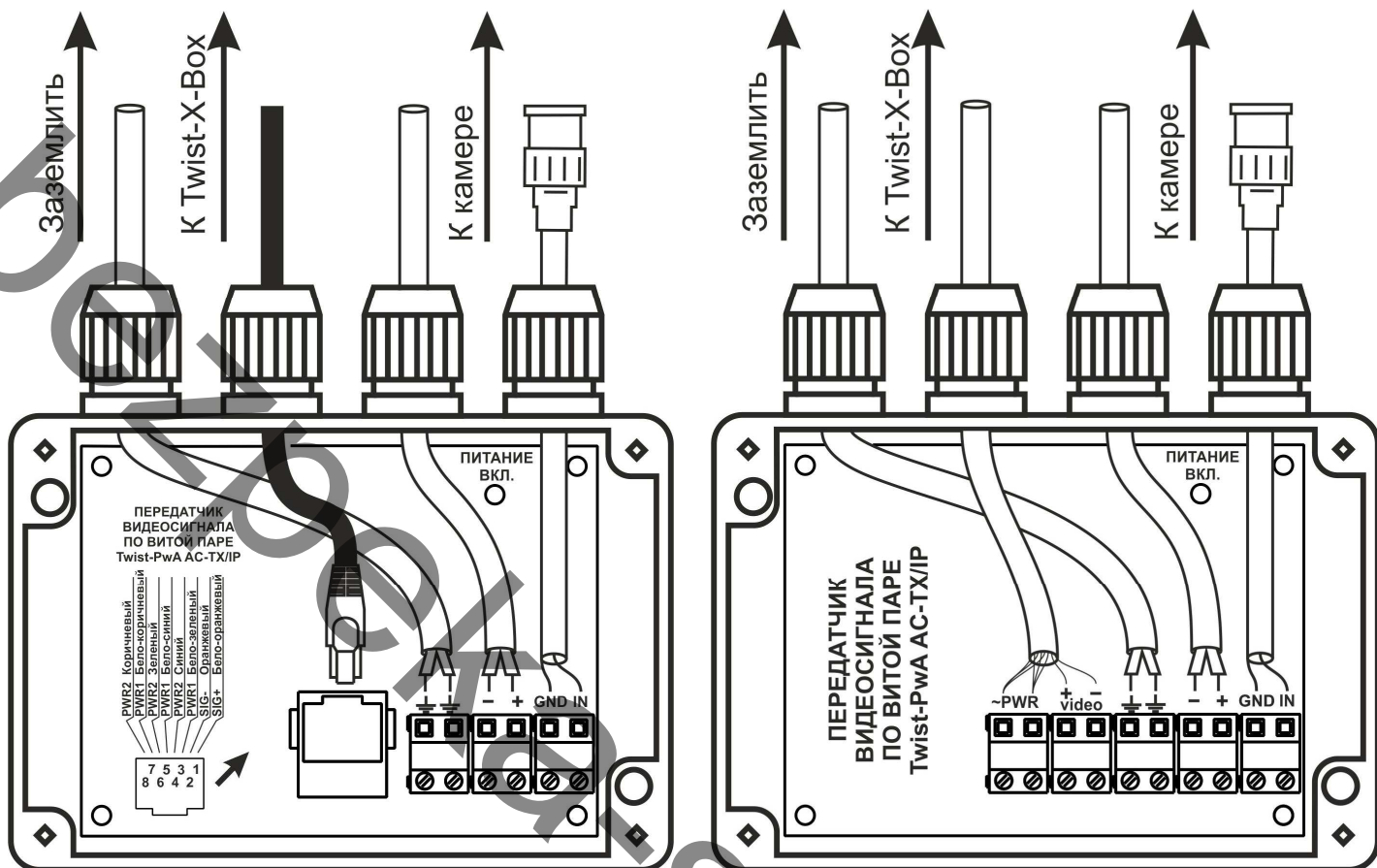
Рис.2 Подключения кодера TWIST-PWA-AC-TX-IP-2A (RJ-45 и клеммник для витой пары)
