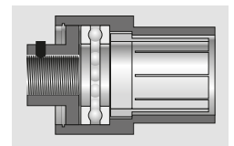
TWTC втулка для вальцевания тонкостенных труб
