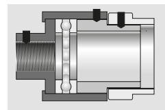
ARTC Регулируемая упорная втулка от 1 до 12 мм
