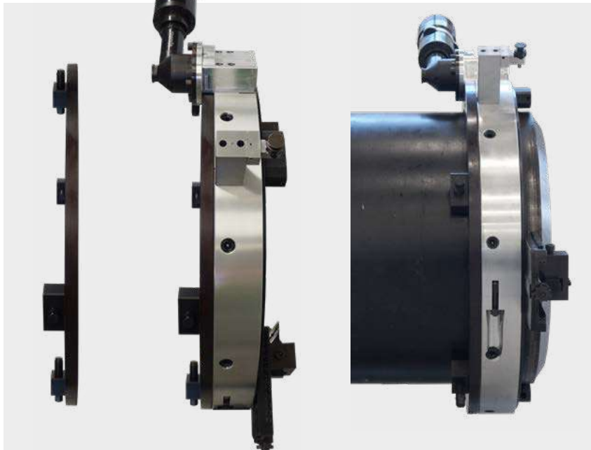
SFSF-1624 с кольцом ORR смонтированным на 24" трубе schedule 120.
