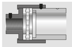
STC Втулка с короткой упорной выемкой глубиной 3 мм. Одинаковая для вальцовок серии 1200 и 800.
