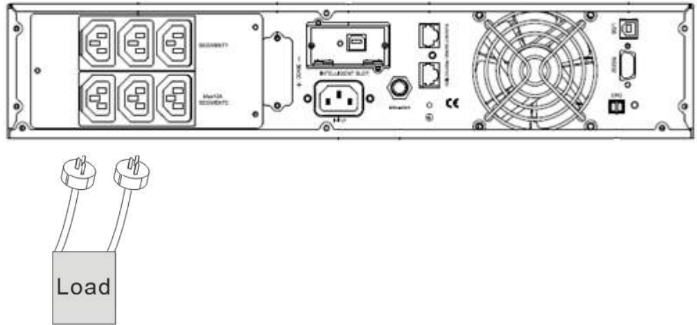
Рис. 7 Подключение нагрузки
