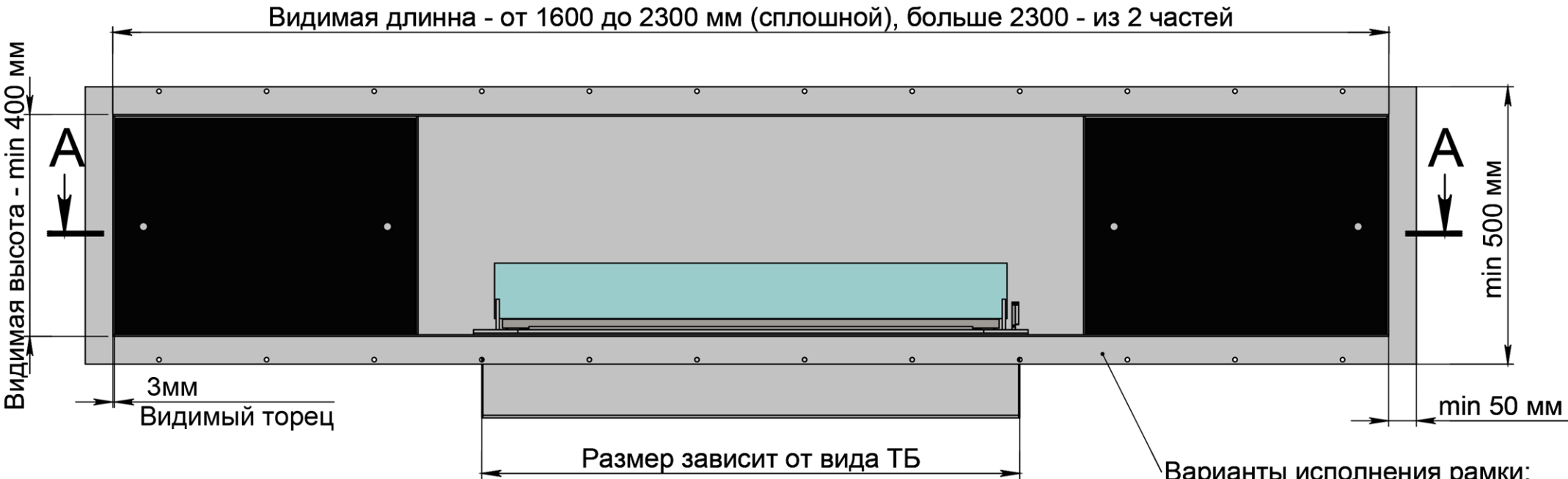
Вид спереди
