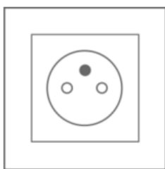
РОЗЕТКА С ЗАЗЕМЛЯЮЩИМ ШТЫРЕМ, ФРАНЦИЯ/БЕЛЬГИЯ
