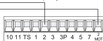
БЛОК УПРАВЛЕНИЯ "SLAVE"
