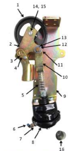
Система натяжки
