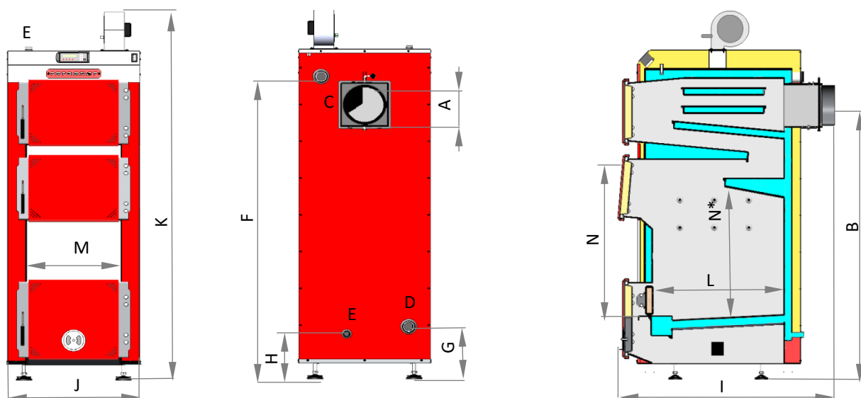
Рис. 6 Габаритні і приєднувальні розміри SPARTAK Uni
