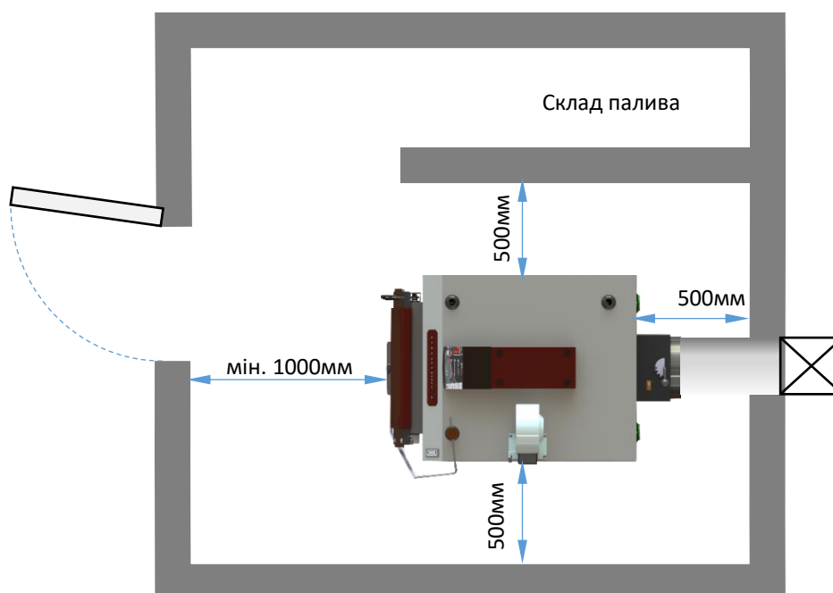
Рис 9 Схема розташування котла в паливній.
