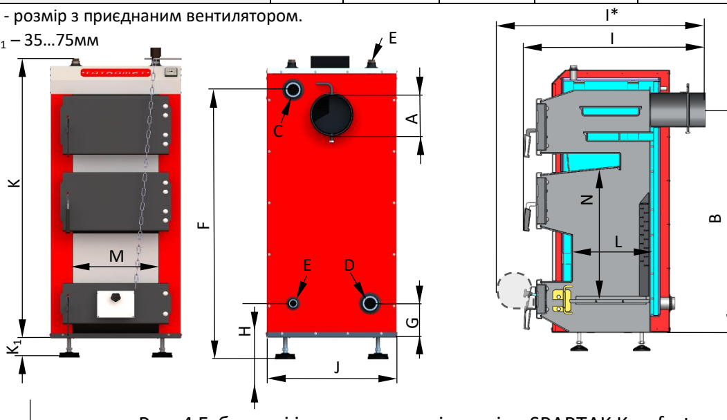
Рис. 4 Габаритні і приєднувальні розміри SPARTAK Komfort
