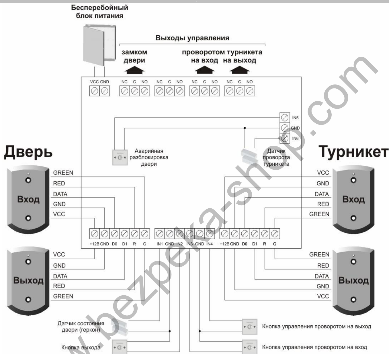
Рис . 4. Вариант подключения NAC-01 для управления дверью и турникетом
