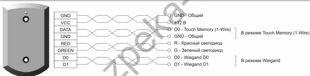
Рис. 2. Подключение считывателей Proximity карт или брелков PR-XX
