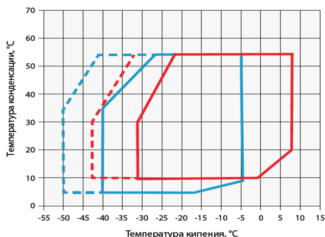
Рабочий диапазон для R404A
