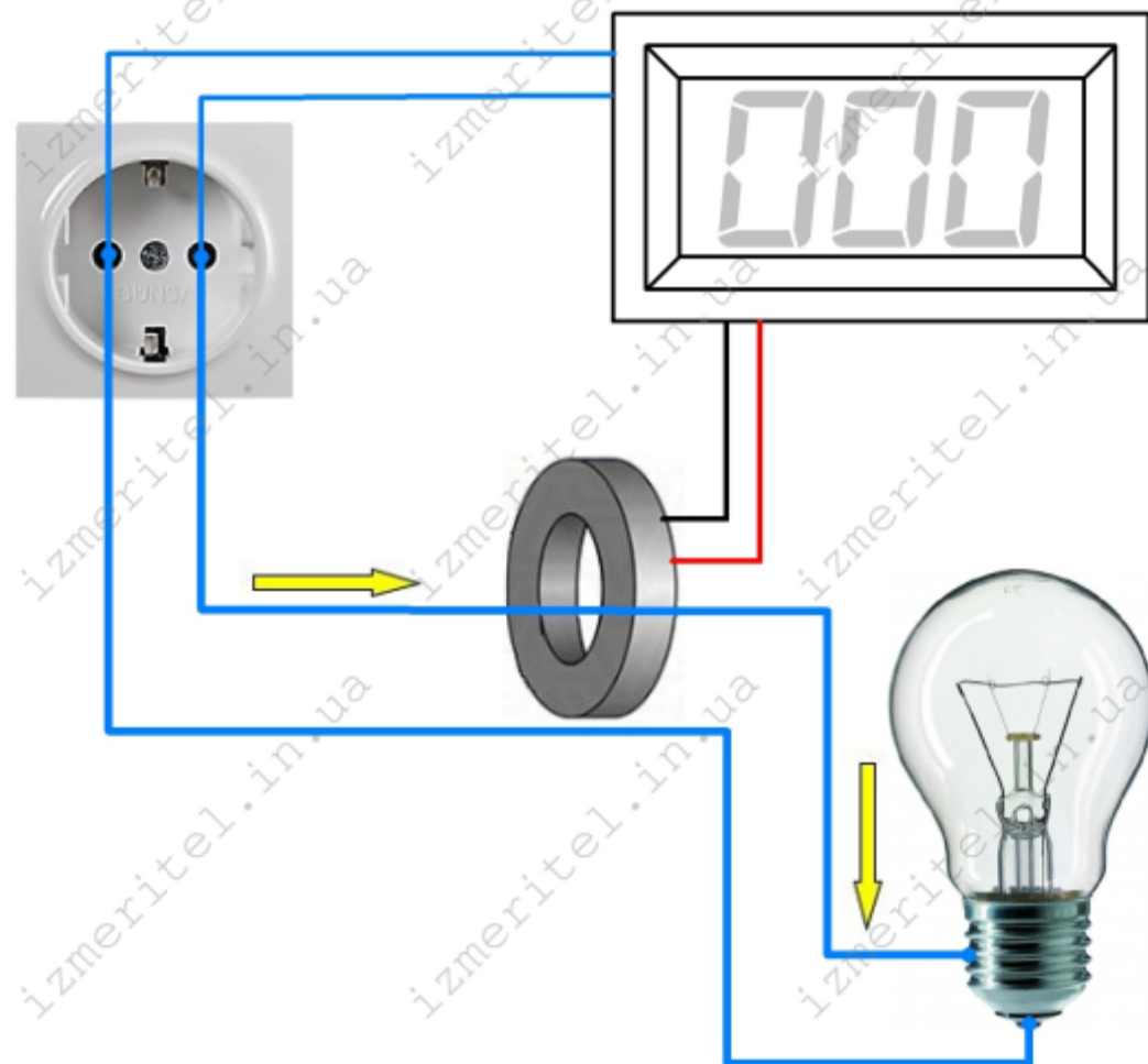
Схема подключения от измеряемого источника питания
