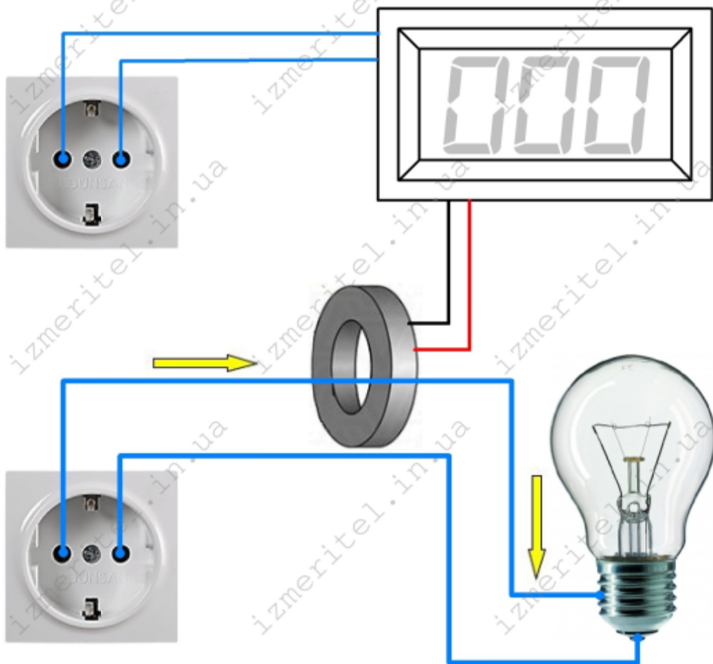
Схема подключения от внешнего источника питания
