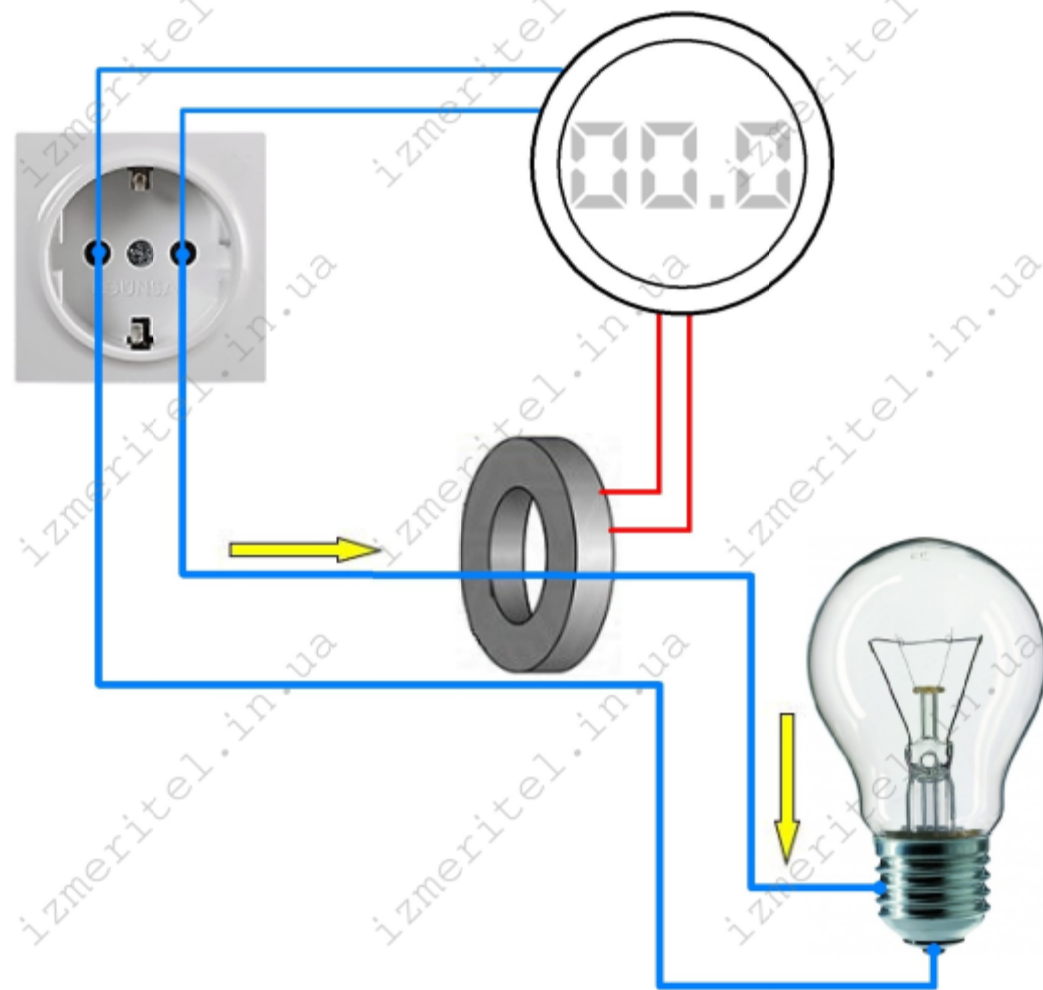
Схема подключения от измеряемого источника питания
