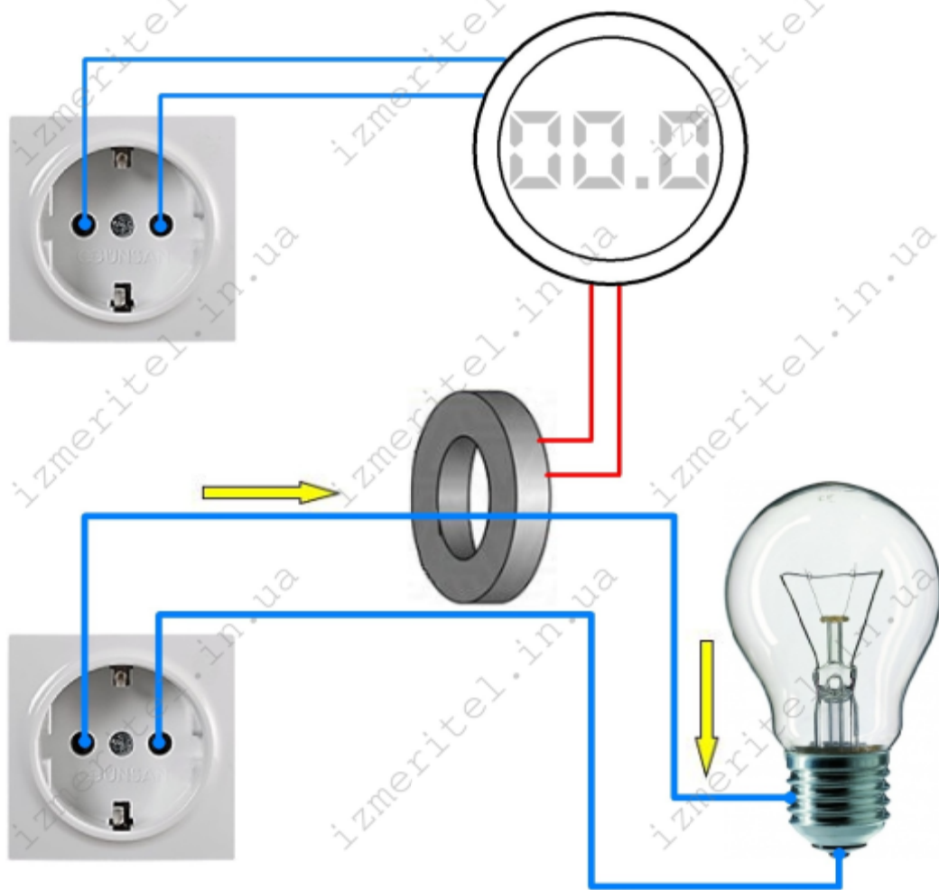
Схема подключения от внешнего источника питания
