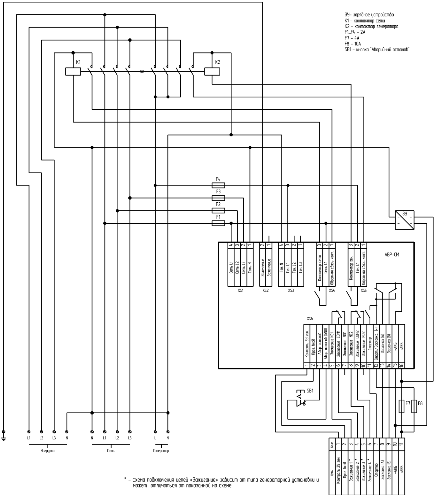
Рис. 6.3. Схема подключения АВР-СМ для конфигурации АВР313 с общим нейтральным проводом
