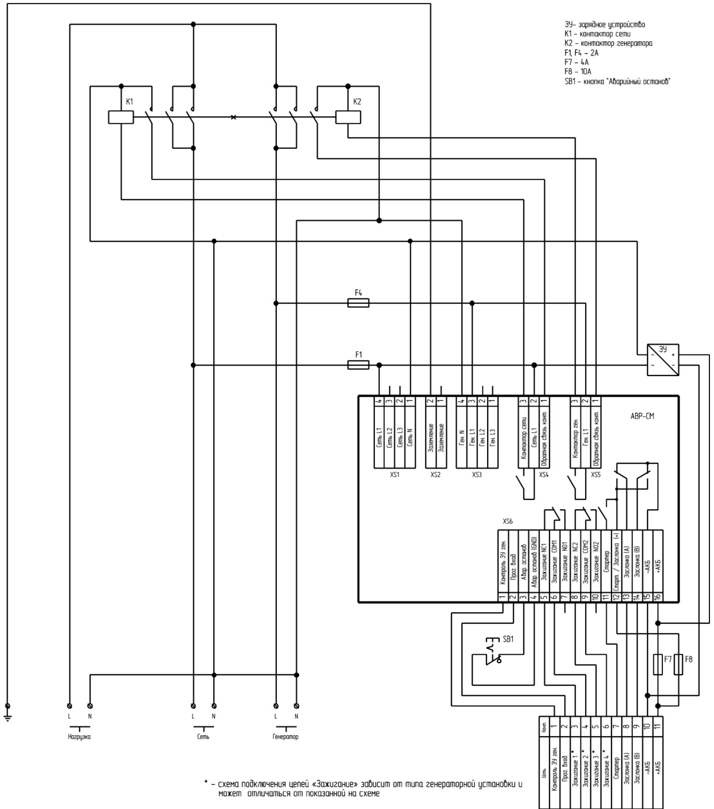
Рис. 6.4. Схема подключения АВР-СМ для конфигурации АВР11 с общим нейтральным проводом
