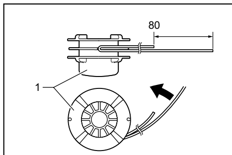
► 1. Spool
