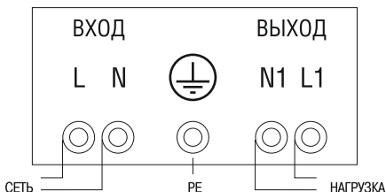
Рис 3. Схема подключения стабилизаторов от 3 до 12 кВА
