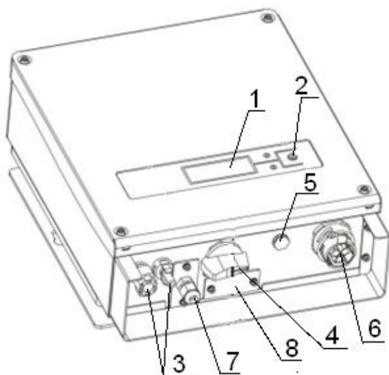
Рисунок 2 – Инвертор
