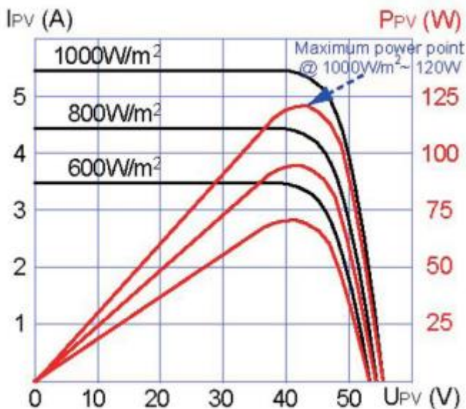
Рисунок 5 – Характеристики солнечной панели.
