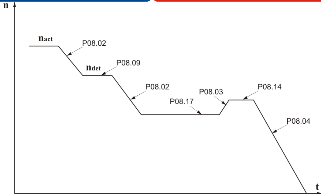
Рисунок 6-6 Временная диаграмма выполнения функции ориентированного торможения
