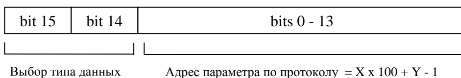
Рисунок 6-16 Структура адресного поля
