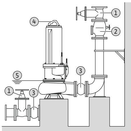
Fig. 8: Установка в непогруженном состоянии
