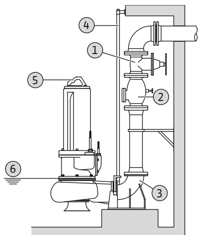
Fig. 6: Стационарная установка в погруженном состоянии
