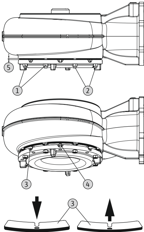
Fig. 13: SOLID G: регулировка зазора
