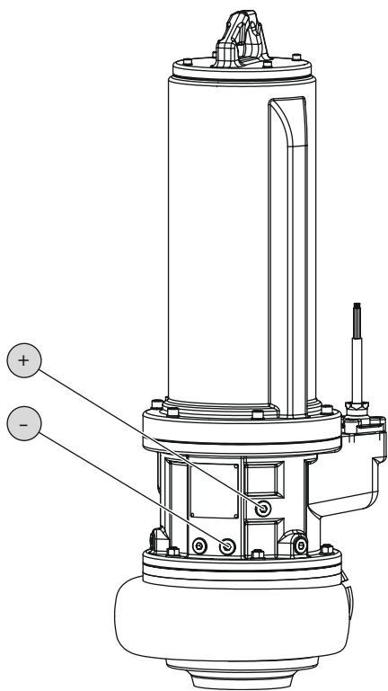
Fig. 5: Камера уплотнений: проверка масла
