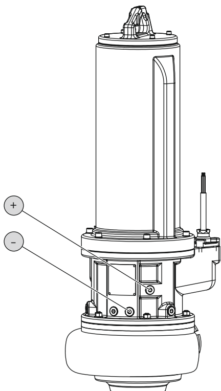
Fig. 11: Камера уплотнений: замена масла
