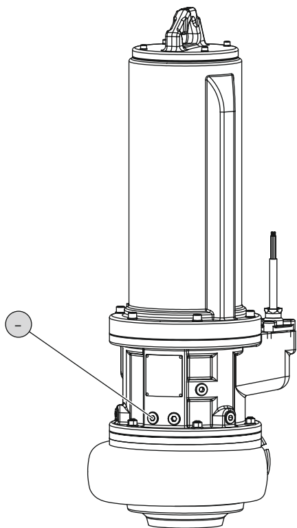
Fig. 9: Опорожнение камеры утечек
