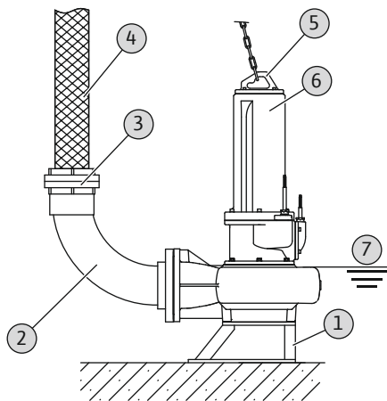
Fig. 7: Переносной вариант установки в погруженном состоянии
