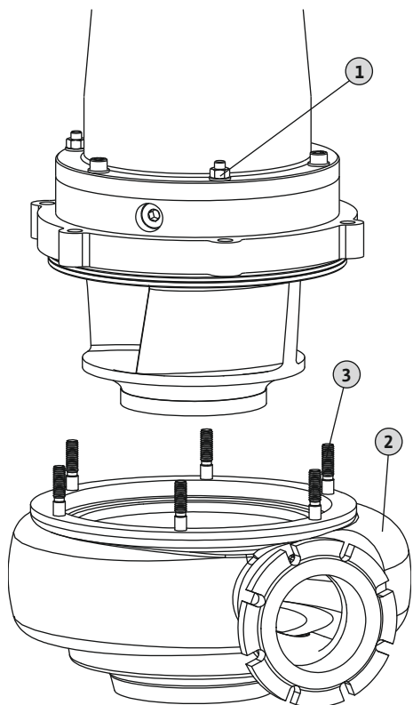
Fig. 12: Замена гидравлического корпуса
