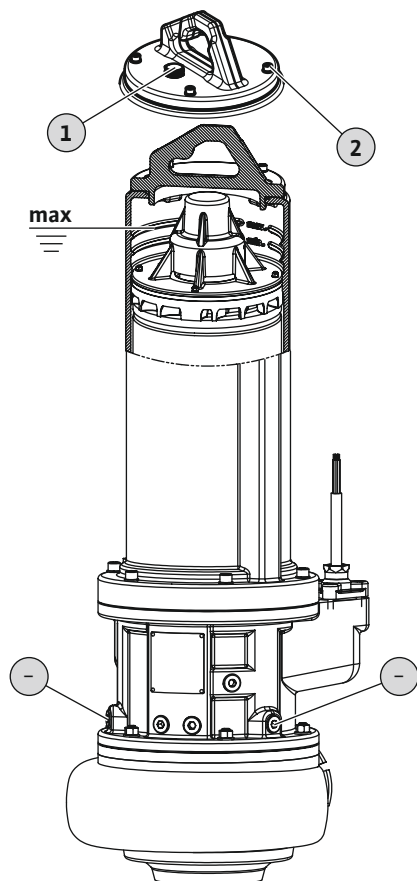
Fig. 4: Проверка охлаждающего средства
