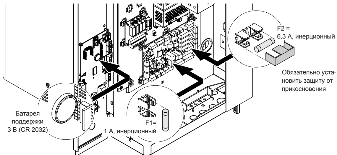
Рис. 6. Положение батареи поддержки и предохранителей на плате привода
