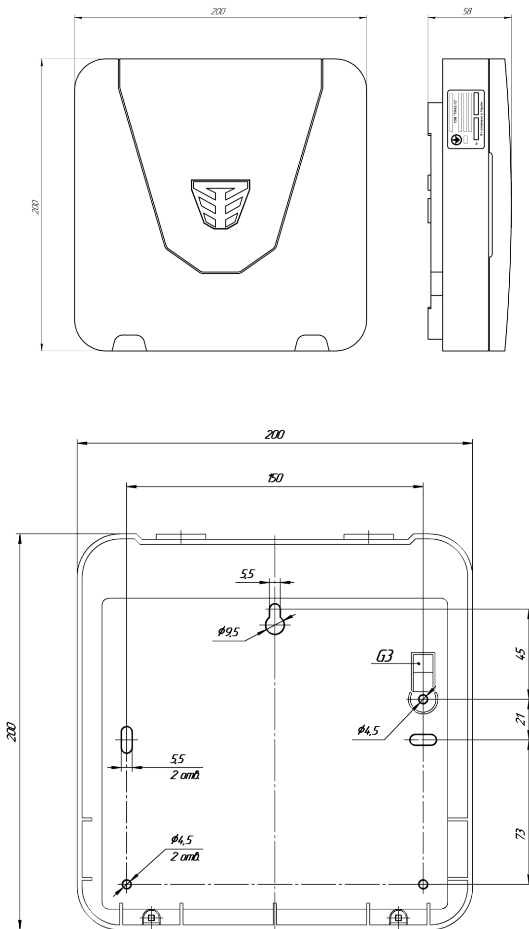
Рисунок Б.1 – Установчі розміри ППК
