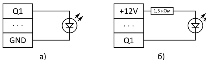
Рисунок 2.6 – Схеми підключення індикаторів підтвердження
