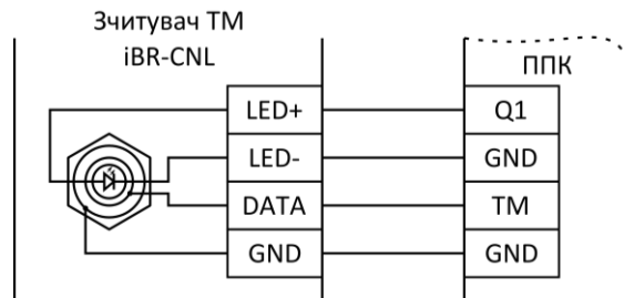
Рисунок 2.7 – Схема підключення зчитувача ключів ТМ
