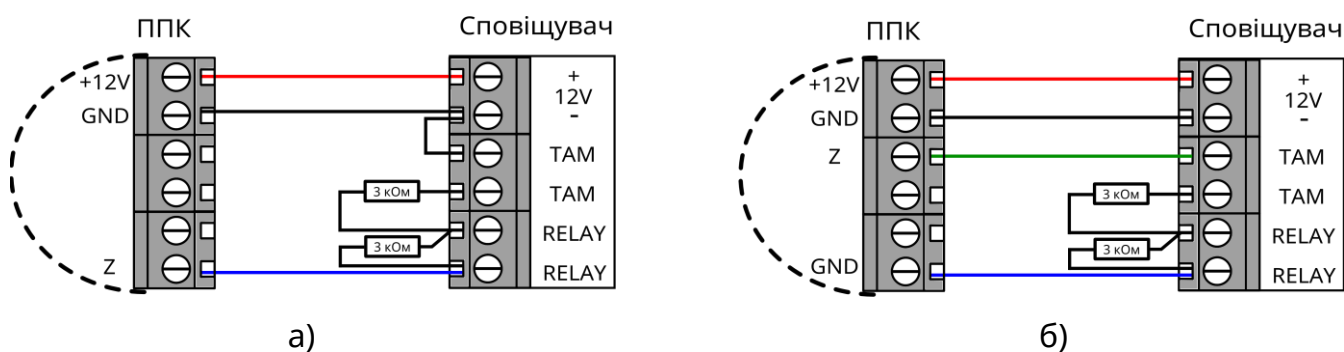
Рисунок 2.4 – Приклади підключення сповіщувачів по типу 2EOL
