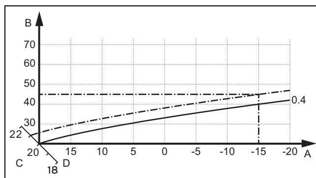
A Зовнішня температура, °C B Задана температура лінії подачі, °C C Задана температура приміщення, °C D Вісь а
