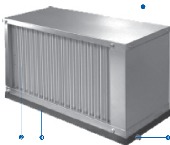
1 корпус, 2 пластины каплеуловителя, 3 ванна для конденсата, 4 система отвода конденсата
