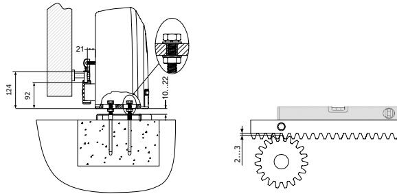
Малюнок 5. Регулювання положення двигуна
