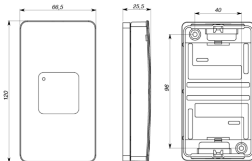
Рис 2. Габаритные размеры
