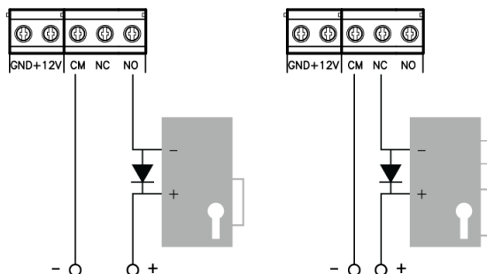
Рис.7. Подключение замков
