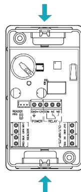
Рис 3. Подвод кабеля
