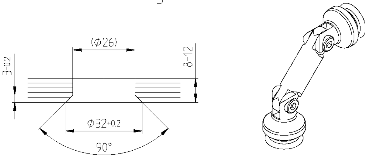
Detail Senkbohrung
