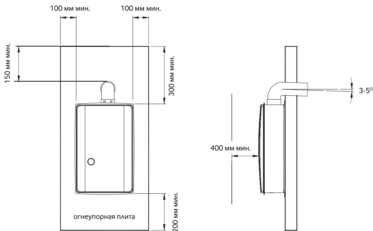
Рисунок 11. Установка котла
