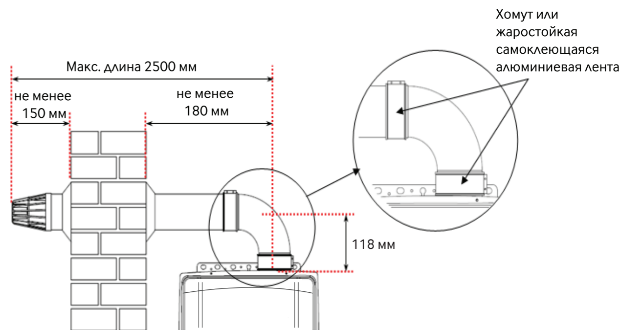
Рисунок 12. Установка дымохода
