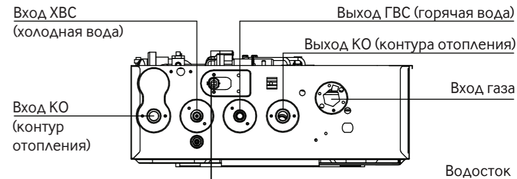
Рисунок 1. Устройство и назначение основных частей
