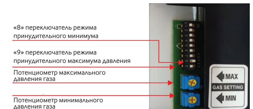
Рисунок 15. DIP-переключатели
