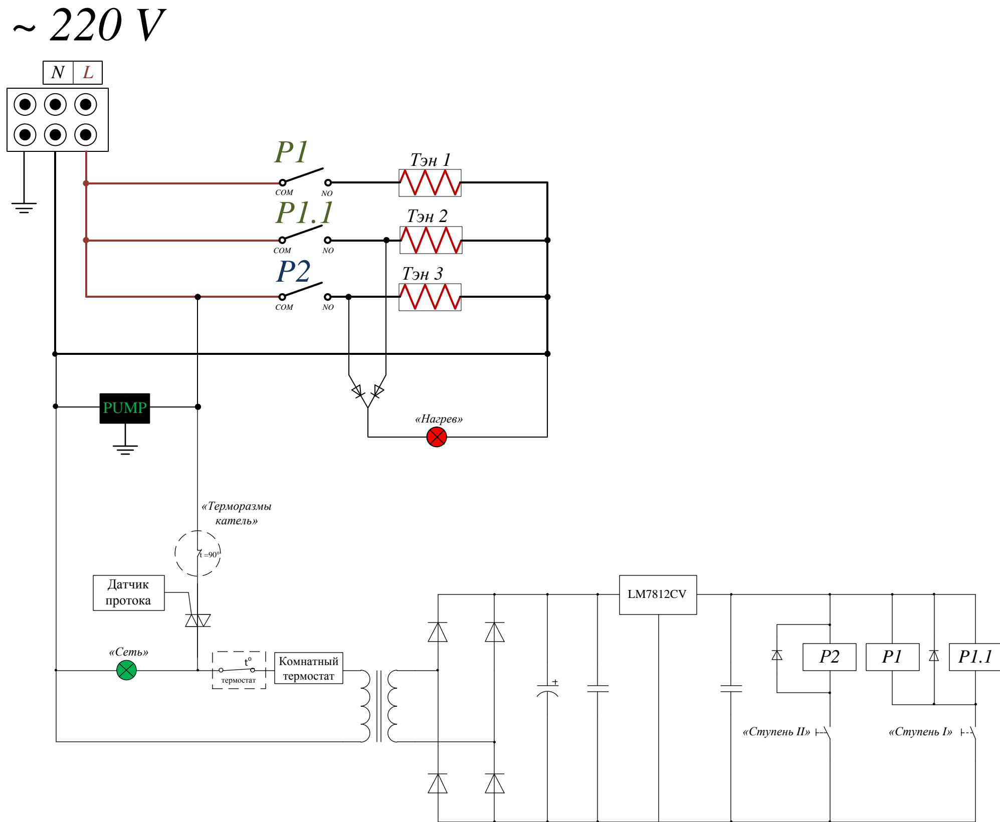
Рисунок 3 – Схема электрическая принципиальная для котлов «Standart» на 220 В
