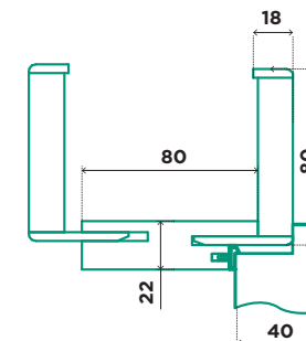
КОРОБКА «БРАМА PROFІ» ЛИШТВА «80» ПОКРИТТЯ «ЕКОЦЕЛ»
