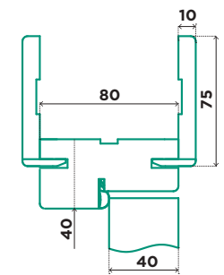
КОРОБКА «ПРЕСТИЖ» ЛИШТВА «НЮАНС»
