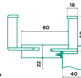
КОРОБКА «БРАМА PROFІ» ЛИШТВА «60» ПОКРИТТЯ «ЛІНІЯ ДЕРЕВА»
