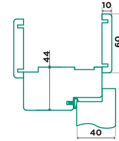
КОРОБКА «СТАНДАРТНА 80» ЛИШТВА «60» ПОКРИТТЯ «ЛІНІЯ ДЕРЕВА» ПОКРИТТЯ «ЕКОЦЕЛ»
